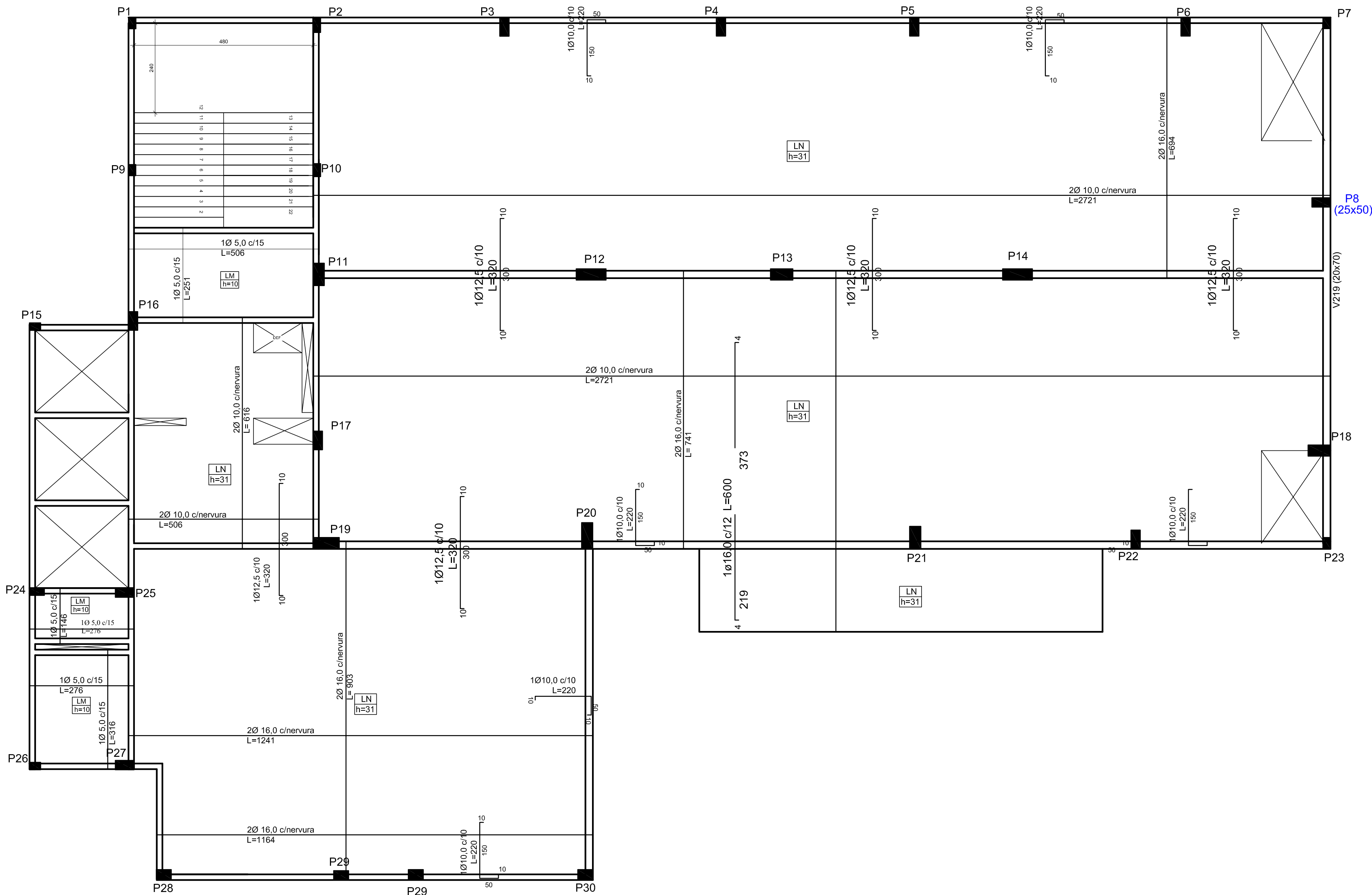
Planta de Fôrmas 3º Pavimento - Ferragem Escala 1:75
